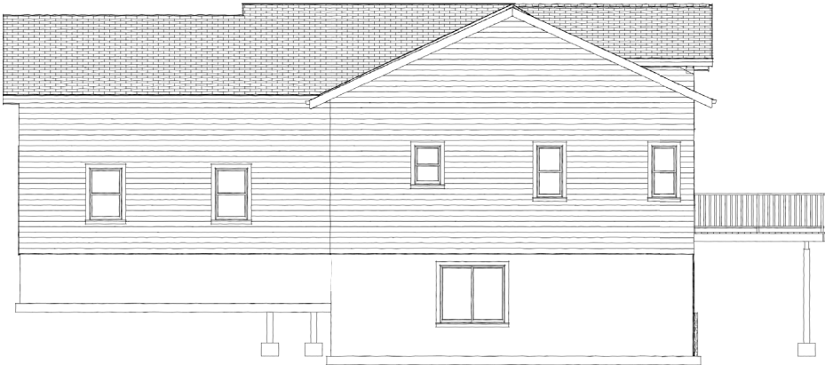
Right Elevation
